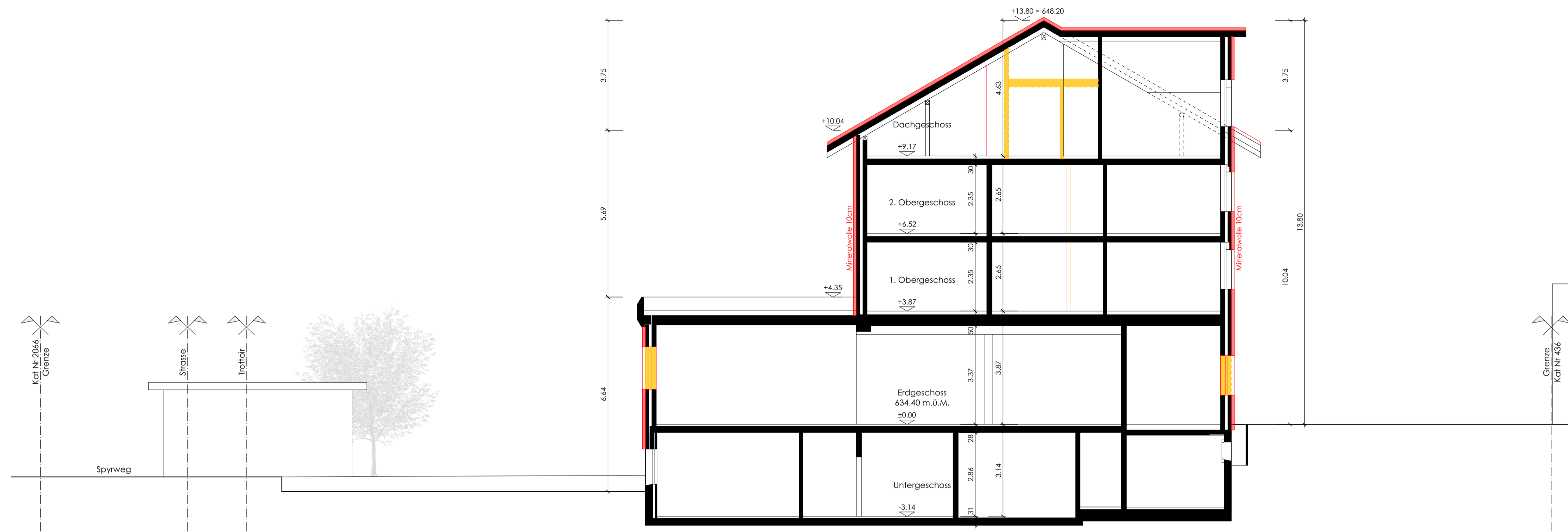
Schnitt A
